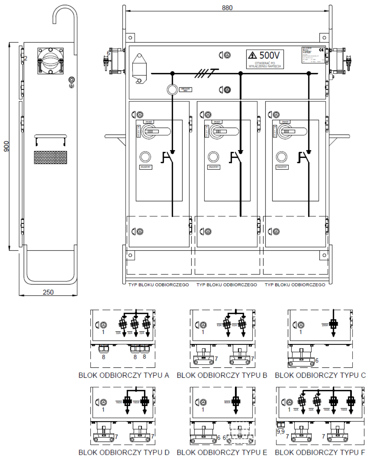
Rys. 1 Widok zewnętrzny zestawu przełotowo-rozdzielczego typu ZPR-05/3
