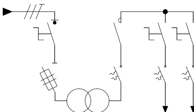
Rys. 2 Schemat jednokreskowy zestawu transformatorowego typu ZT-05/1,6/2
