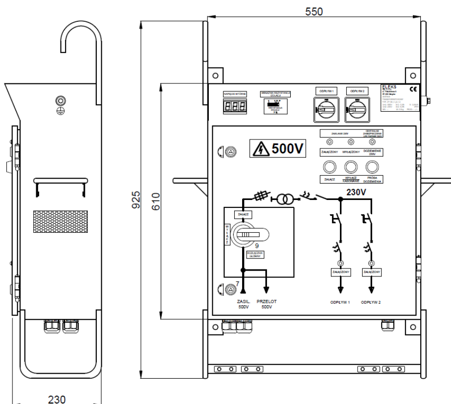
Rys. 1 Widok zewnętrzny zestawu transformatorowego typu ZT-05/1,6/2
