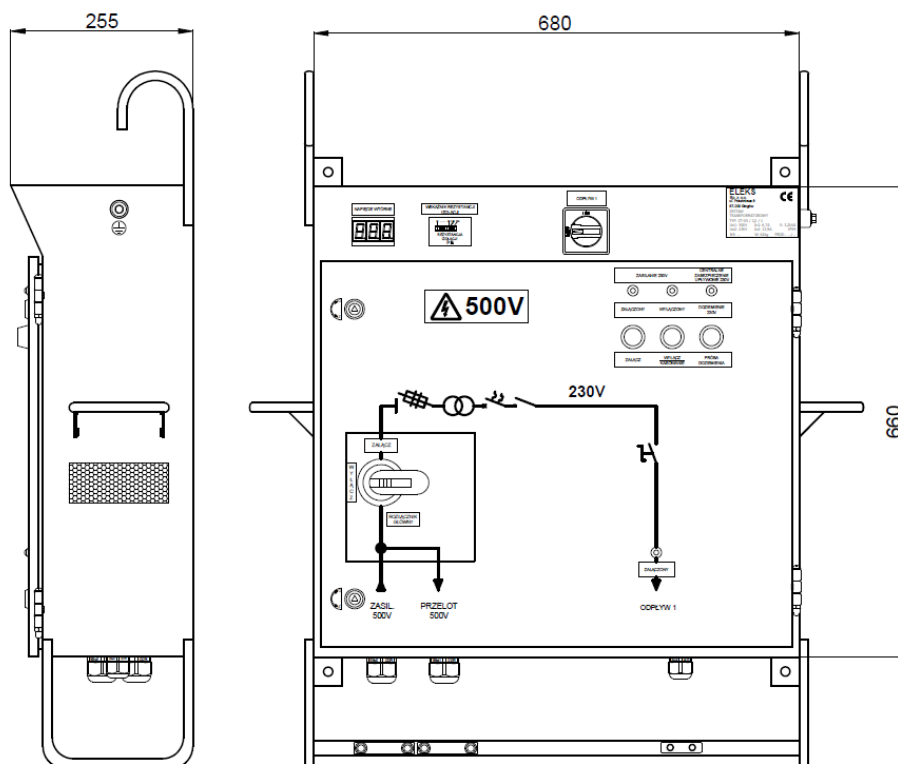
Rys. 1 Widok zewnętrzny zestawu transformatorowego typu ZT-05/3,2/1
