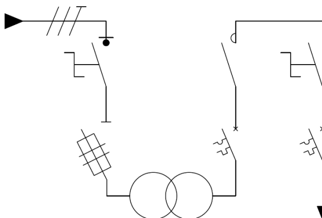
Rys. 2 Schemat jednokreskowy zestawu transformatorowego typu ZT-05/3,2/1
