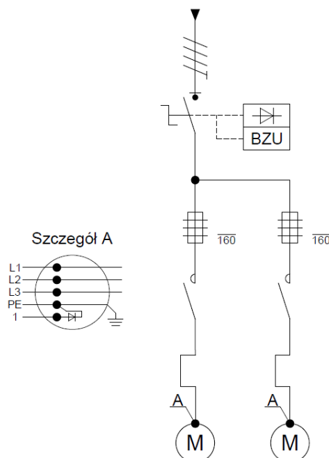
Rys. 2 Schemat jednokreskowy zestawu zasilającego niskonapięciowego typu ZZN-05/2x30kW
