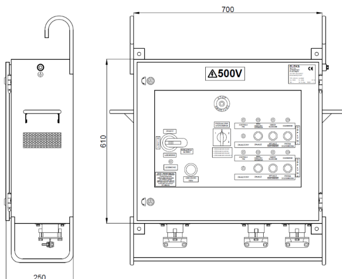
Rys. 1 Widok zewnętrzny zestawu zasilającego niskonapięciowego typu ZZN-05/2x30kW
