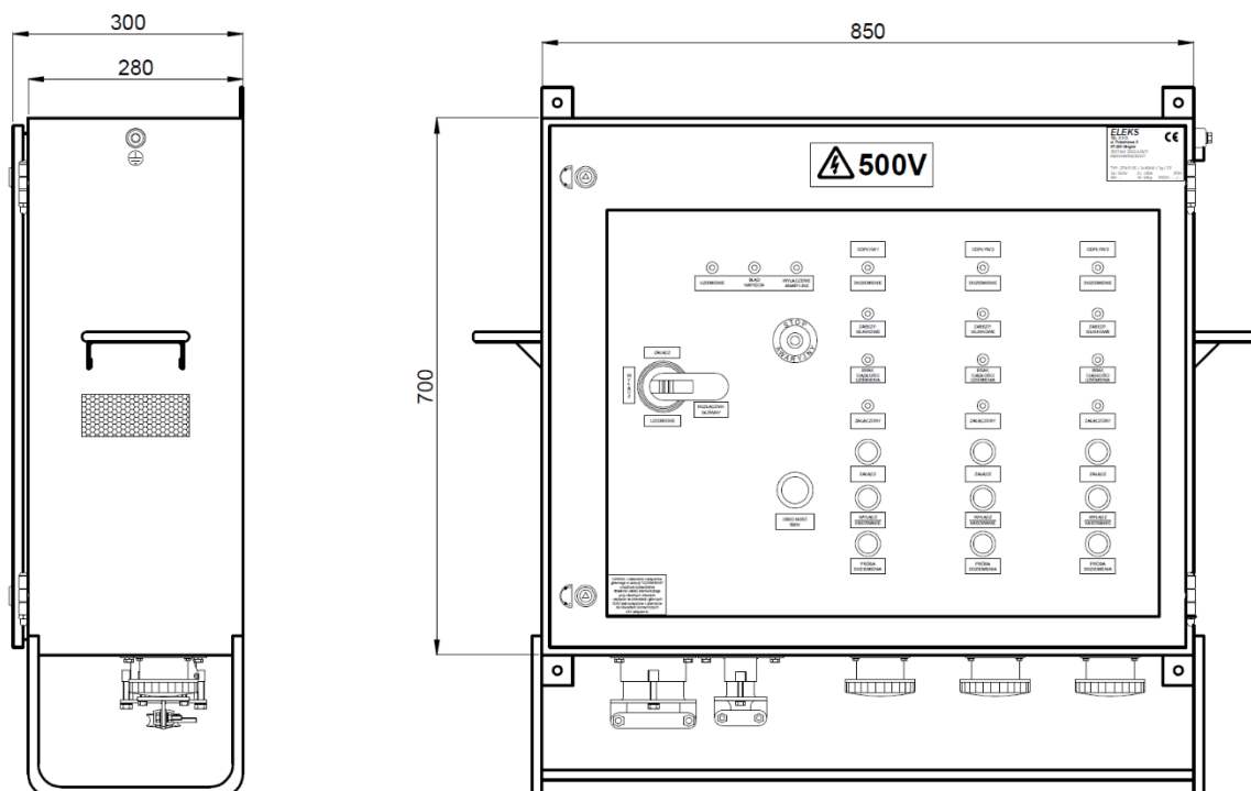
Rys. 1 Widok zewnętrzny zestawu zasilającego niskonapięciowego typu ZZN-P-05/3x40kW/3g/ZP
