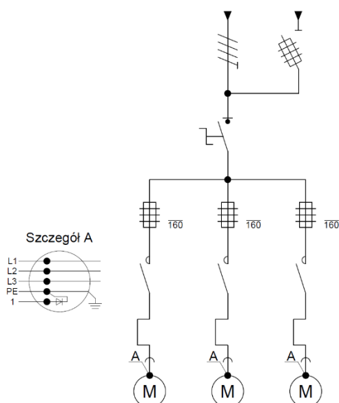
Rys. 2 Schemat jednokreskowy zestawu zasilającego niskonapięciowego typu ZZN-P-05/3x40kW/3g/ZP
