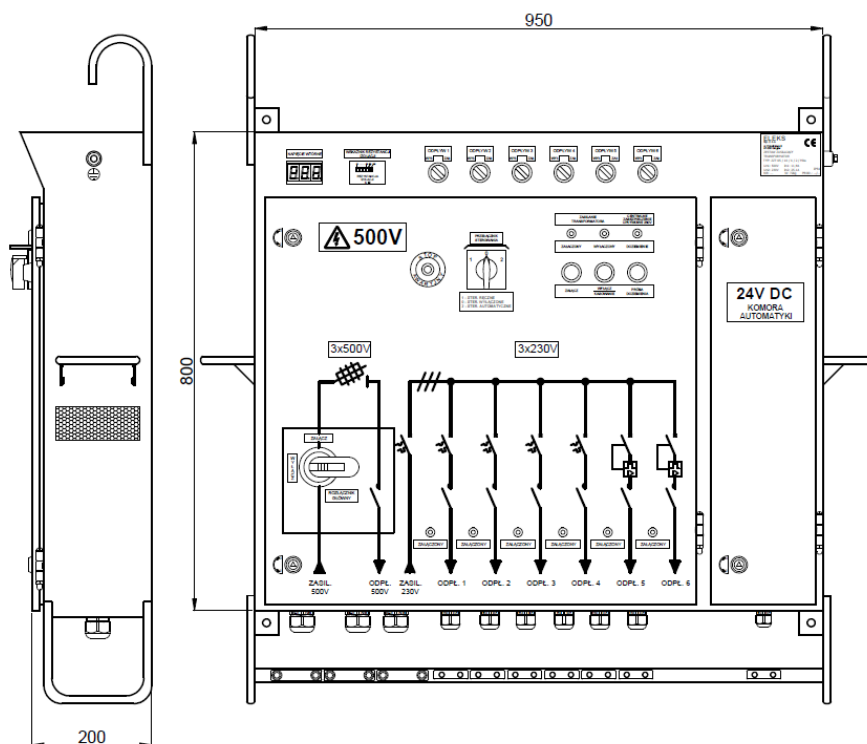
Rys. 1 Widok zewnętrzny zestawu zasilającego transformator typu ZZT-05/10/4/2/Mbs
