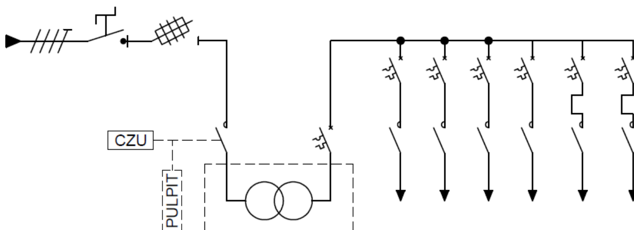
Rys. 2 Schemat jednokreskowy zestawu zasilającego transformator typu ZZT-05/10/4/2/Mbs
